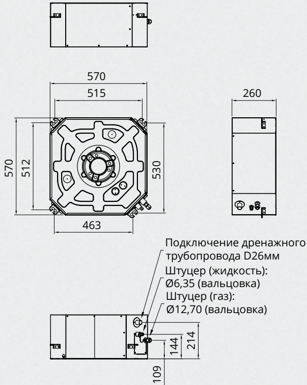
Модели: ALCA-H18/4DR1A
