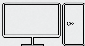
Программное обеспечение
