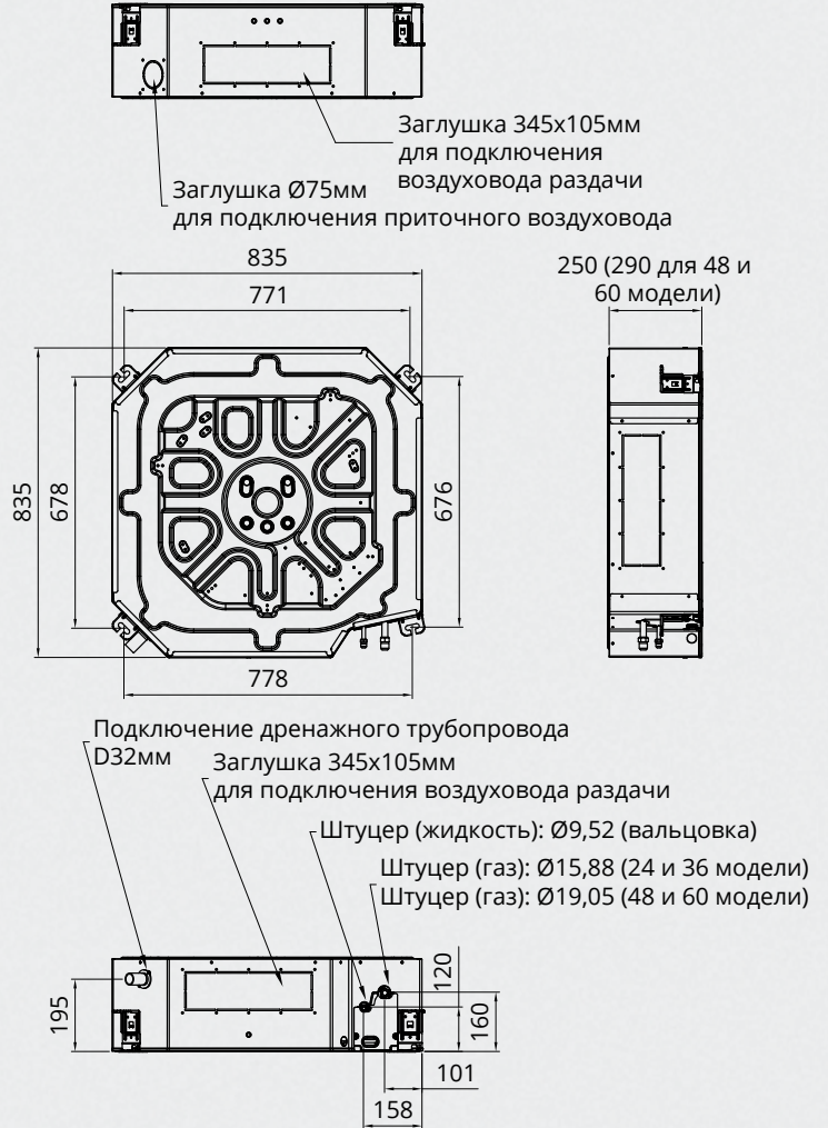
Модели: ALCA-H24(36/48/60)/4DR1
