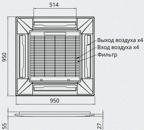
Модель: MB12
